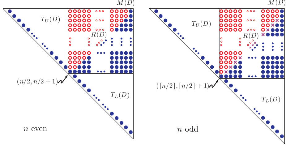
Figure 7: The regions T_U(D) , R(D) , and T_L(D) .
